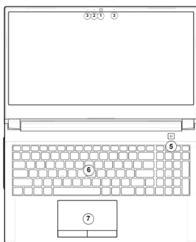
Figura 4 - Vista frontal con la pantalla abierta
