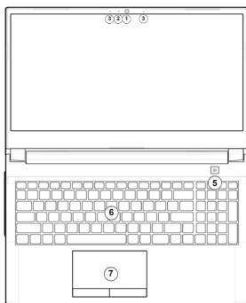
Figura 4 - Vista frontale con schermo aperto
