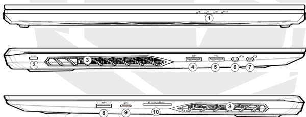
Figura 5 - Visualizzazioni anteriori, di sinistra e di destra
