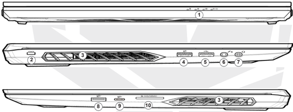
Şekil 5 - Önden, Soldan ve Sağdan Görünümler
