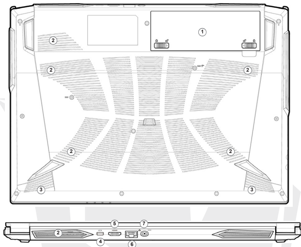
Figura 6 - Vues du bas et de l'arrière
