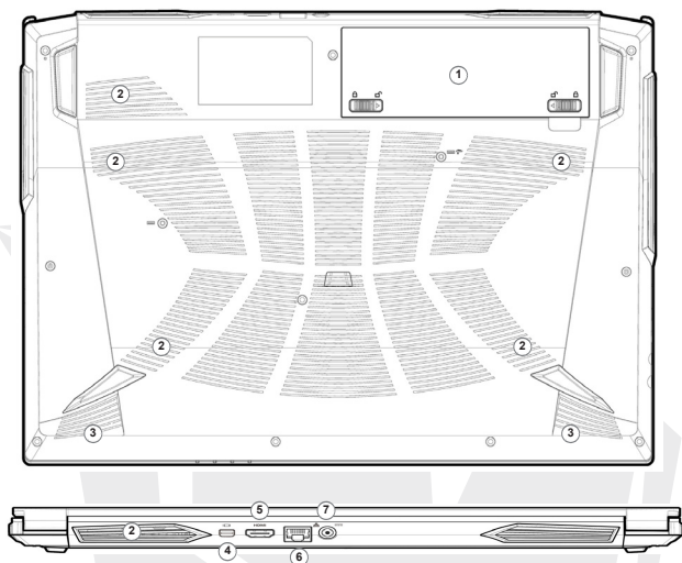
Figura 6 - Visualizzazione inferiore e posteriore
