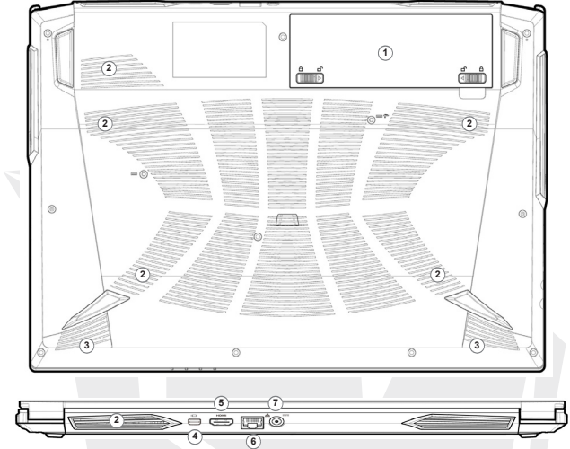
Şekil 6 - Alttan ve Arkadan Görünümler
