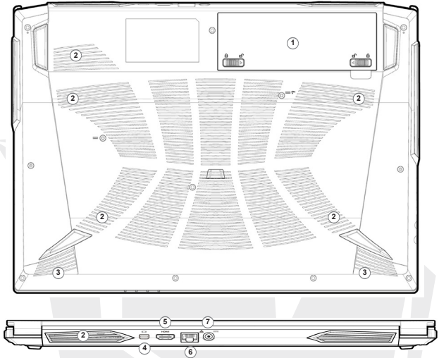
الشكل 7 الشكل من الأسفل والخلف
